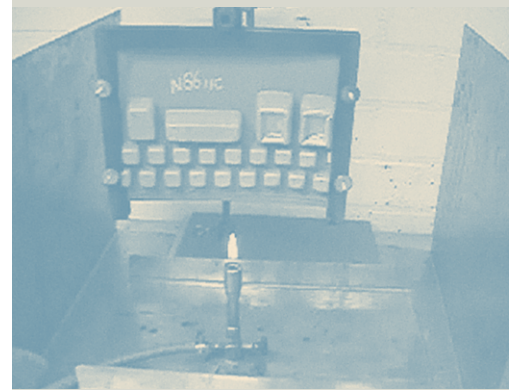
Prova di combustione secondo PV3357
